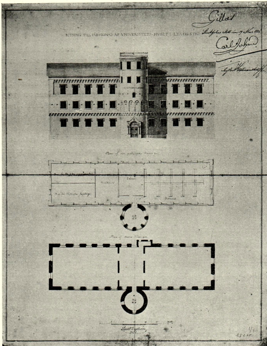
FIG. 21. A. NYSTRÖM: FÖRSLAG TILL PÅBYGGNAD AV AKADEMIHUSET, GILLAT AV KONUNGEN ÅR 1836. (U. A.)
