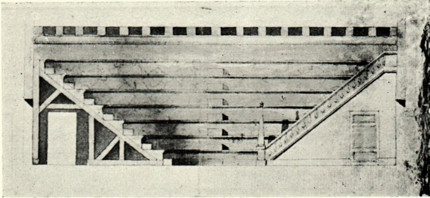
FIG. 8. C. HÄRLEMAN: RITNING TILL ANATOMISK TEATER VID AKADEMIEN I LUND. (U. A.)
