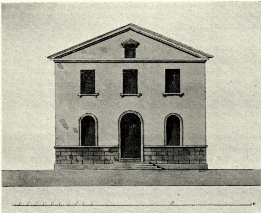
FIG 18. C. F. Sundwall: RITNING TILL FLYGELBYGGNAD (KUGGIS) VID AKADEMIEN. (Kungl. Byggnadsstyrelsen.)
