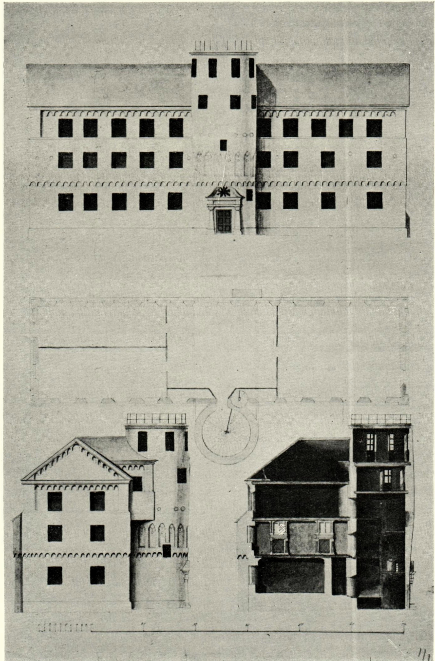
FIG. 19. C. F. HILL: FÖRSLAG TILL PÅBYGGNAD AV AKADEMIHuset. (R. A.)
